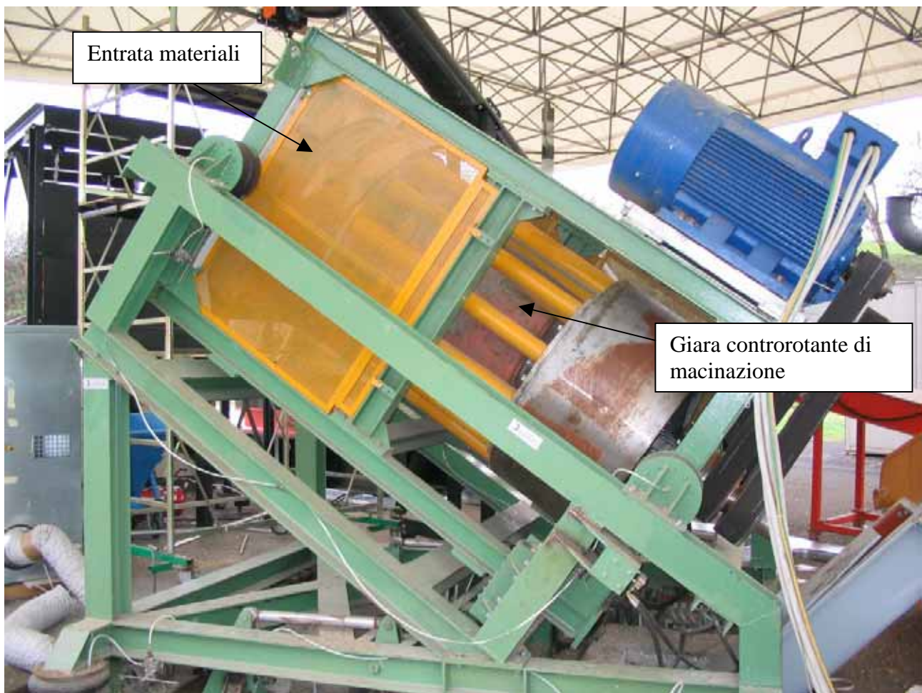
Figura 6: Immagine del mulino a nutazione nell'impianto pilota di Montelibretti (capacità di trattamento 2 ton/ora)
