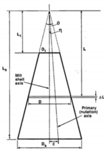
Figura 1: Parametri geometrici di un mulino a nutazione (da D. Hoyer, 1985); lo schema si riferisce a mulini conici del tipo Hicom ( www.hicom-mill.com )
