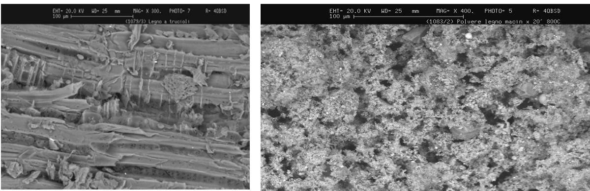
Figura 5: Legno tal quale e sottoposto a micronizzazione (microscopia elettronica a scansione)
